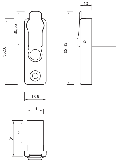
DIMENSIONI ELEMENTO DI RISCONTRO (quote in mm)
